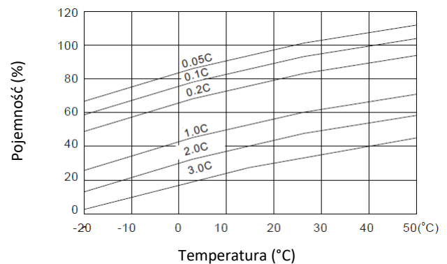
Wpływ temperatury na pojemność
