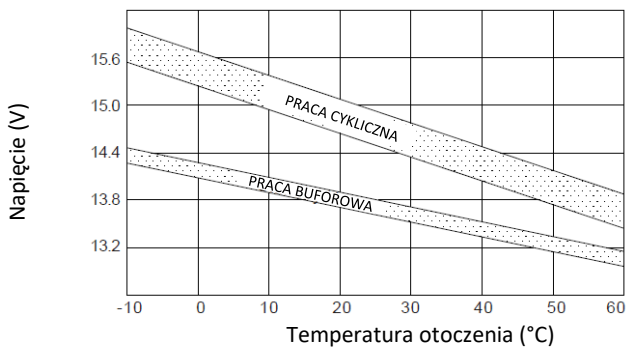
Relacja między napięciem ładowania a temperaturą
