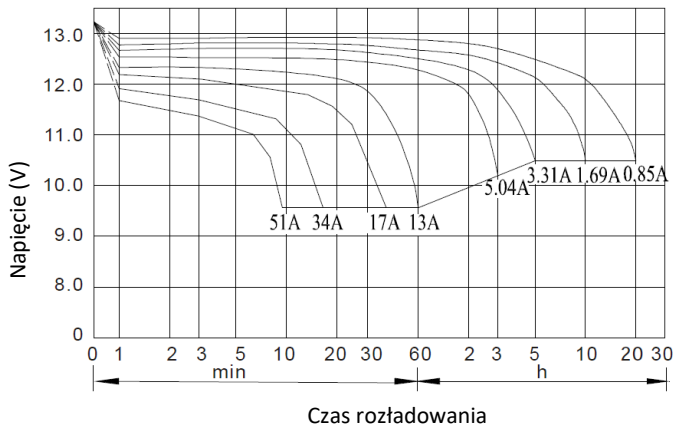
Charakterystyka rozładowania (25°C)
