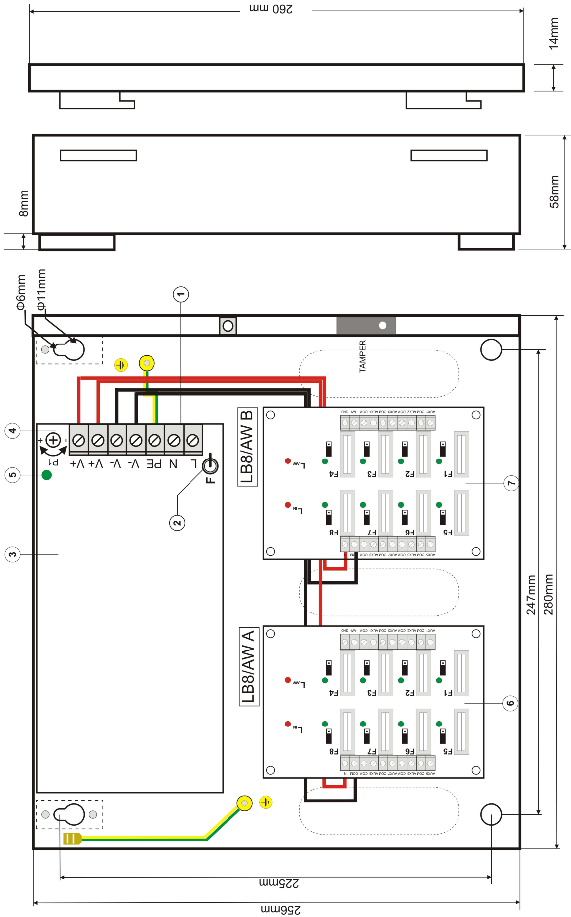
Rys.3. Widok zasilacza.
