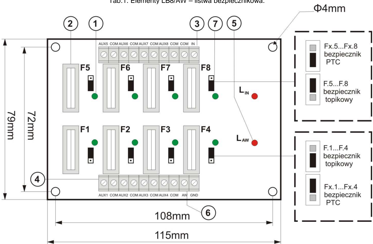
Rys.2. Widok listwy LB8/AW.
