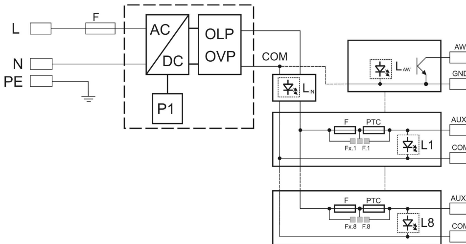
Rys.1. Schemat blokowy zasilacza.
