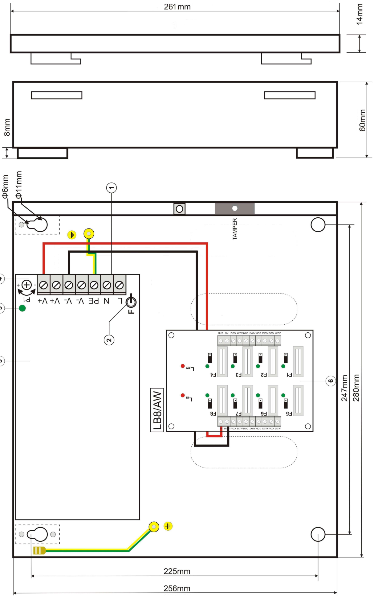
Rys.3. Widok zasilacza.
