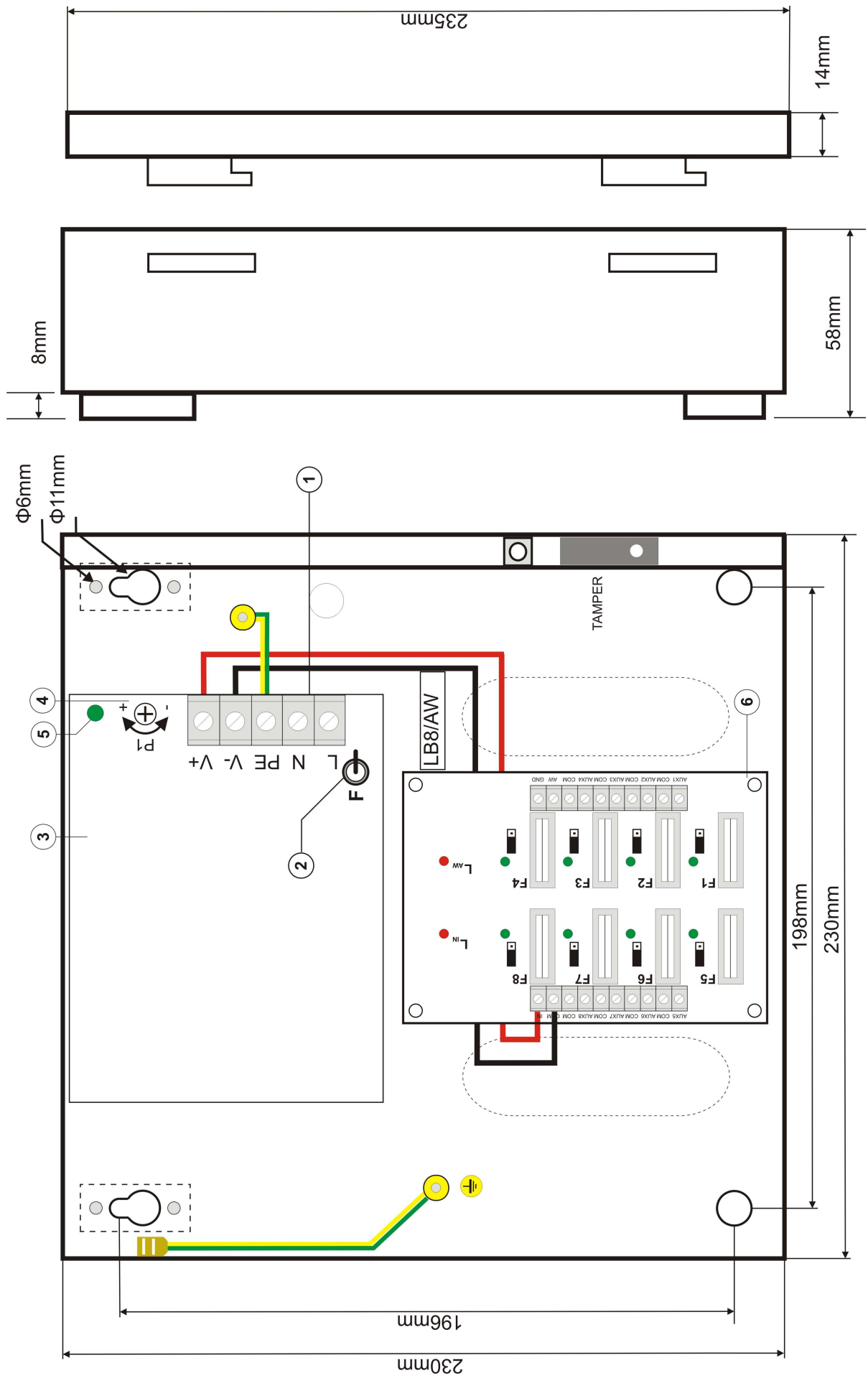
Rys.3. Widok zasilacza.
