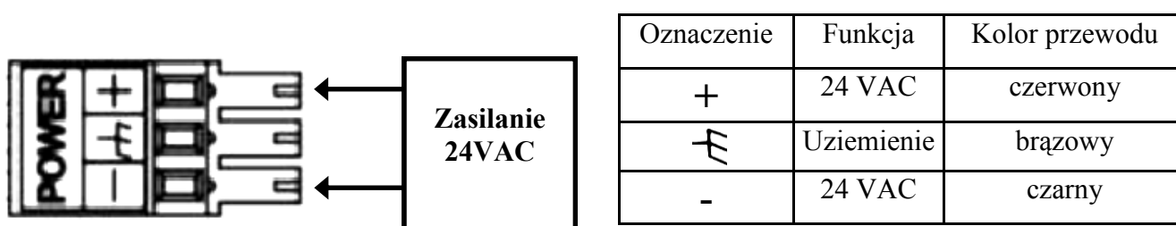
Schemat podłączenia zasilania 24 VAC
