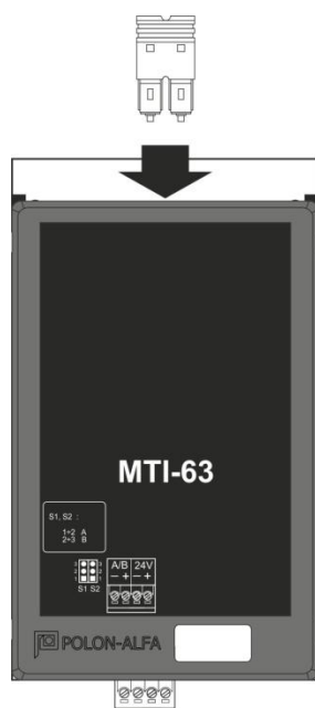
Rys. 23.8.3/1 Moduł MTI-63 – wtyczka typu SC
