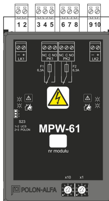
Rys. 7.7/1 Moduł MPW-61
