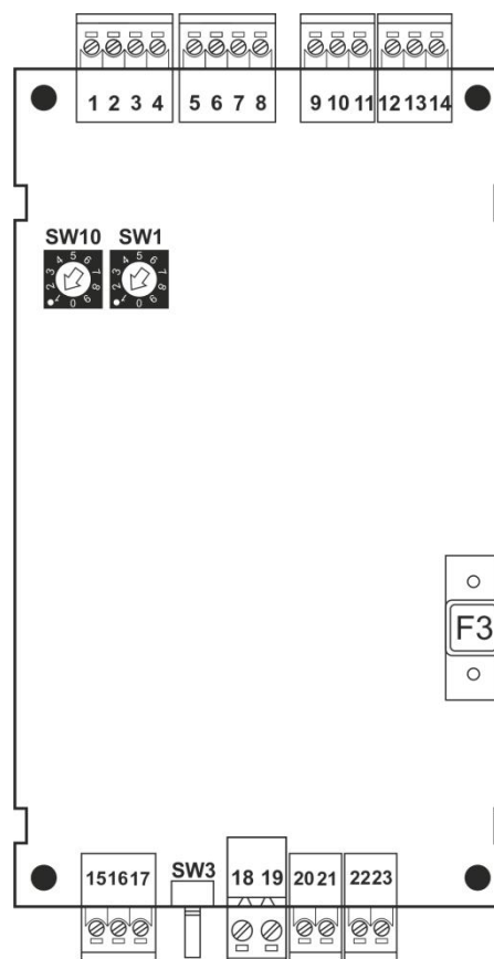
Rys. 8.1/2 Moduł MZP-60
