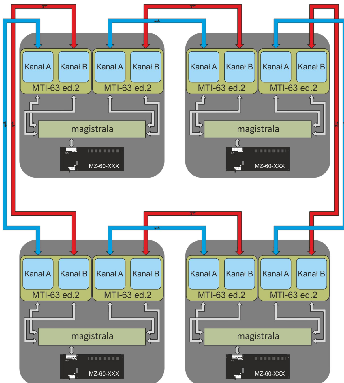
Rys. 23.8.3/5 Połączenie światłowodowe MTI-63 Ed.2 – pierścień (podwójny ring)
