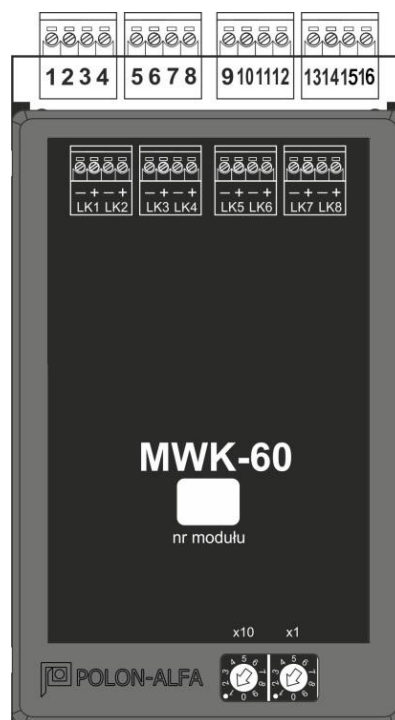
Rys. 7.6/1 Moduł MWK-60
