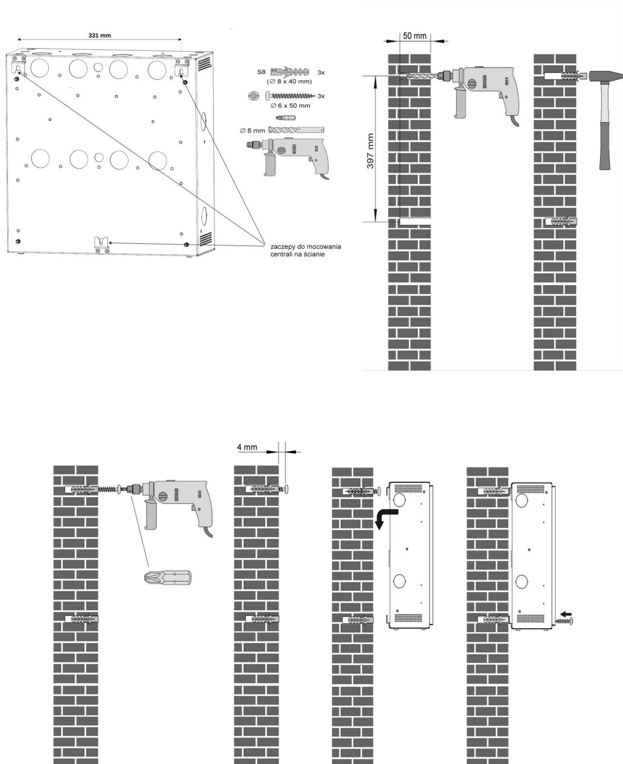
Rys. 23.2/1 Montaż centrali na ścianie – kolejne etapy
