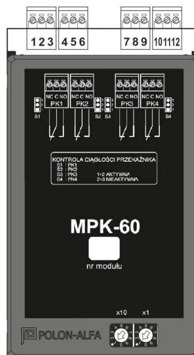
Rys. 7.4/1 Moduł MKS-60
