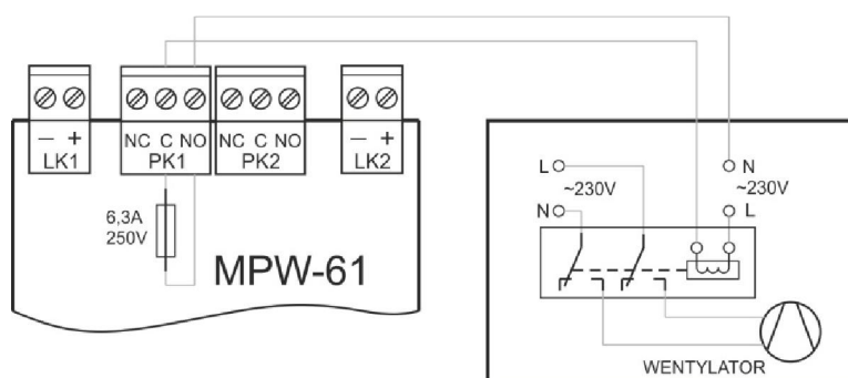
Rys. 7.7/2 Moduł MPW-61
