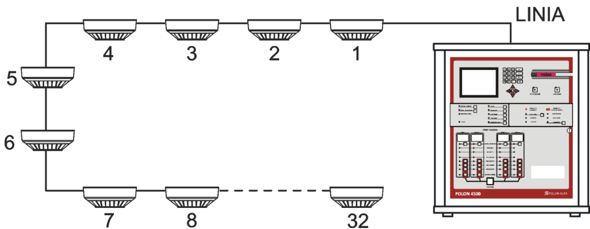
Rys. 6.1 Przykłady adresowalnych linii dozorowych w centrali POLON 4500
