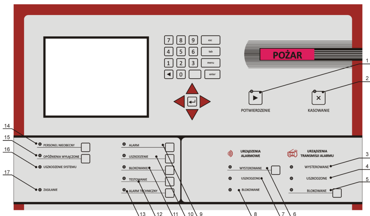
Rys. 4.3 Sygnalizatory optyczne LED bloku wykrywania
