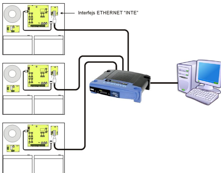
Rys. 29. Komunikacja Ethernet z wykorzystaniem interfejsu Ethernet „INTE”.
