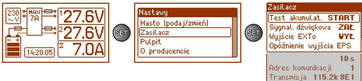
Rys. 25. Ekran „Zasilacz”.
