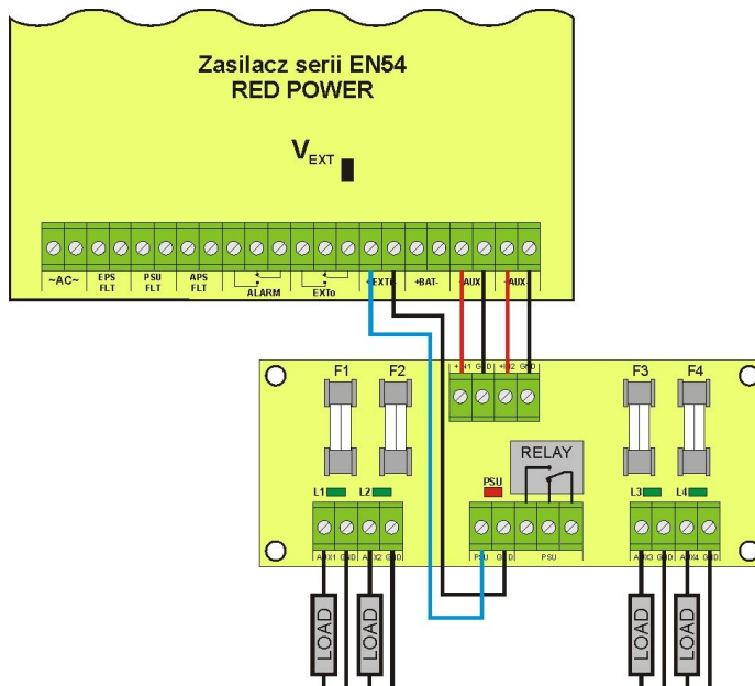
Rys. 21. Sposób podłączenia modułu bezpiecznikowego.
