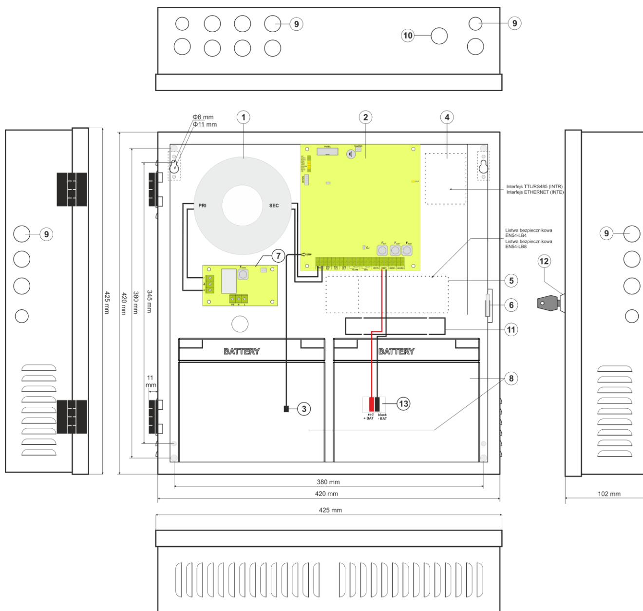
Rys.4. Widok zasilacza.
