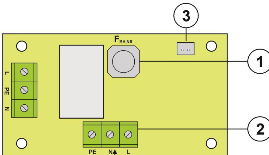
230V Rys. 3. Widok płyty filtra EMC.
