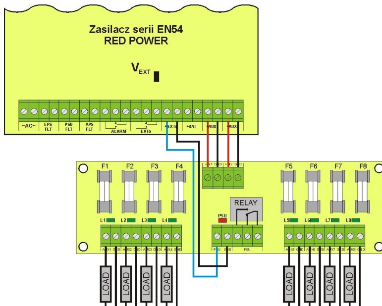
Rys. 20. Przykładowy sposób podłączenia z listwą bezpiecznikową EN54-LB8.
