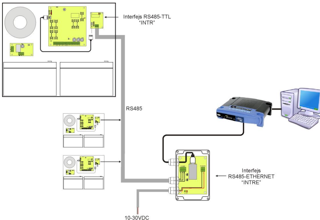
Rys. 30. Komunikacja Ethernet z wykorzystaniem interfejsu RS485-Ethernet „INTE”.
