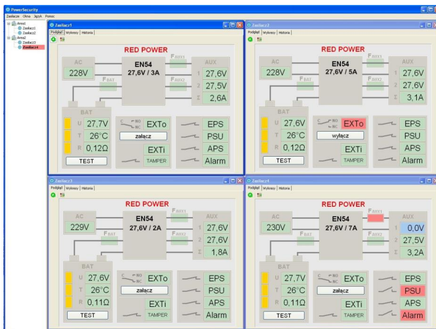
Rys. 31. Panel główny programu „Power security”.
