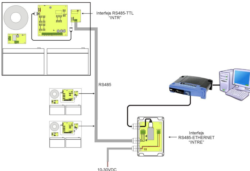
Rys. 30. Komunikacja Ethernet z wykorzystaniem interfejsu RS485-Ethernet „INTRE”.
