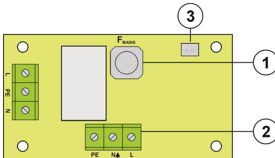
Rys. 3. Widok płyty filtra EMC.
