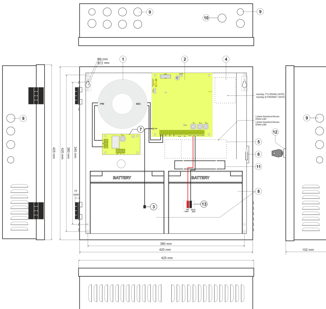
Rys.4. Widok zasilacza.
