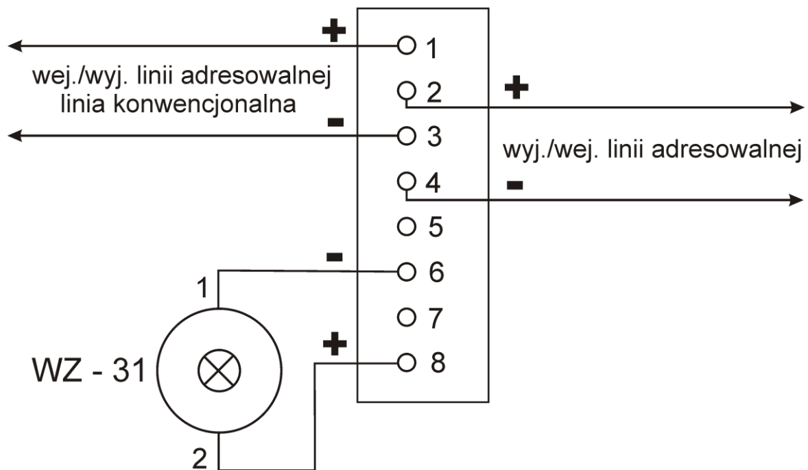
Rys 4. Podłączenie przewodów instalacyjnych do czujki DOP-6001
