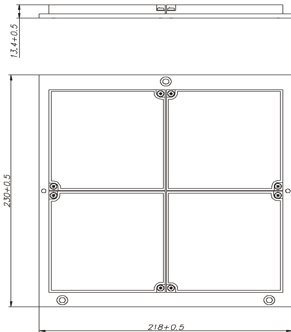
Rys 8. Zespół reflektorów
